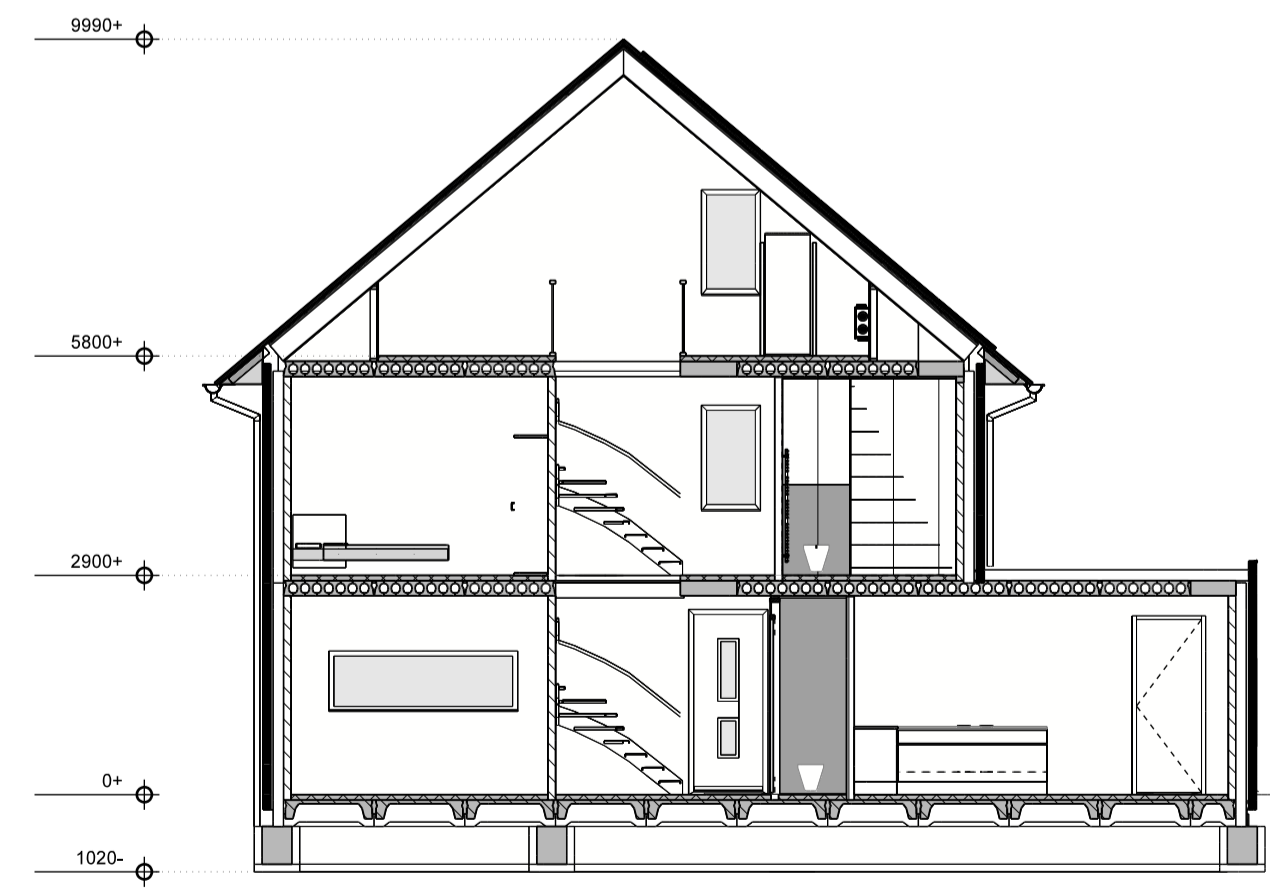
Doorsnede
